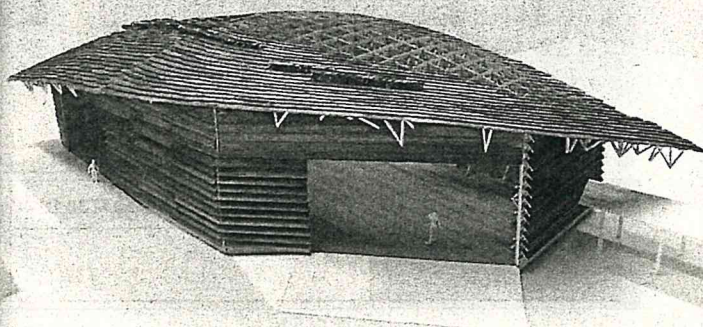
建築概要／木造レシプロカル構造、延べ面積約600㎡
